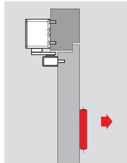
Kozijndorpelmontage tegenscharnierzijde
