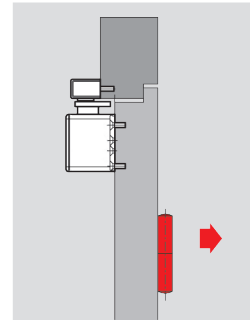
Deurbladmontage tegenscharnierzijde
