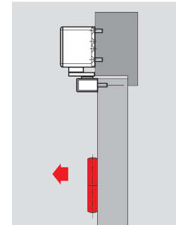
Kozijndorpelmontage scharnierzijde
