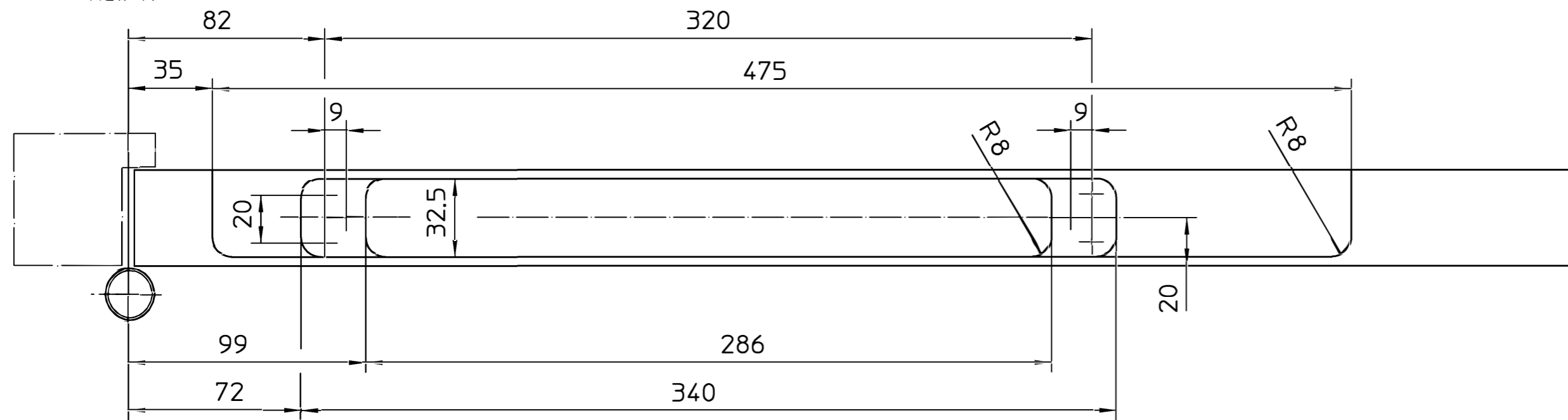
Türblattbearbeitung Door leaf working Ansicht X View X
