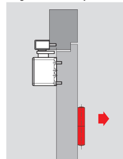
Deurbladmontage tegenscharnierzijde
