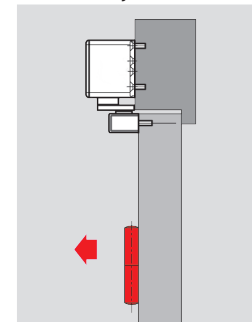
Kozijndorpelmontage scharnierzijde
