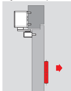
Kozijndorpelmontage tegenscharnierzijde
